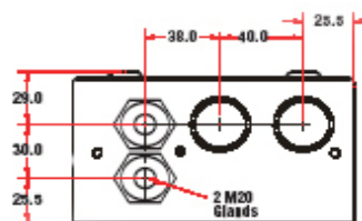
Dimensioner for kabinet med udgang for returluft
